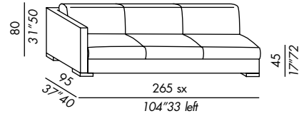
terminale divano letto / end unit sofa bed 265
